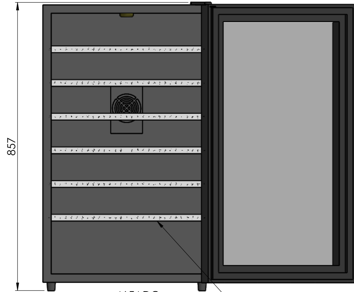
ALZADO
