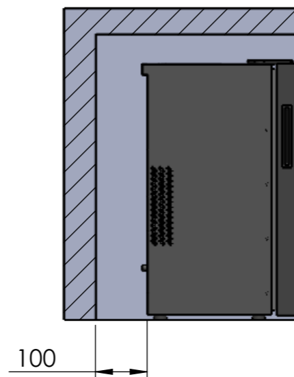
SECCIÓN B-B
