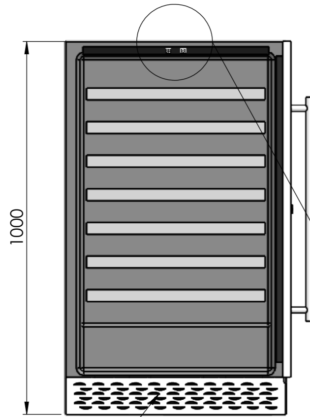
ALZADO
