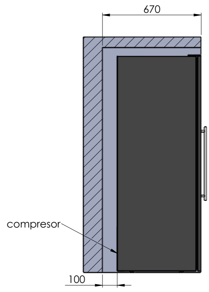
SECCIÓN B-B
