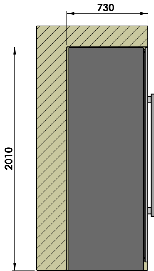
SECCIÓN B-B ESCALA 1 : 20
