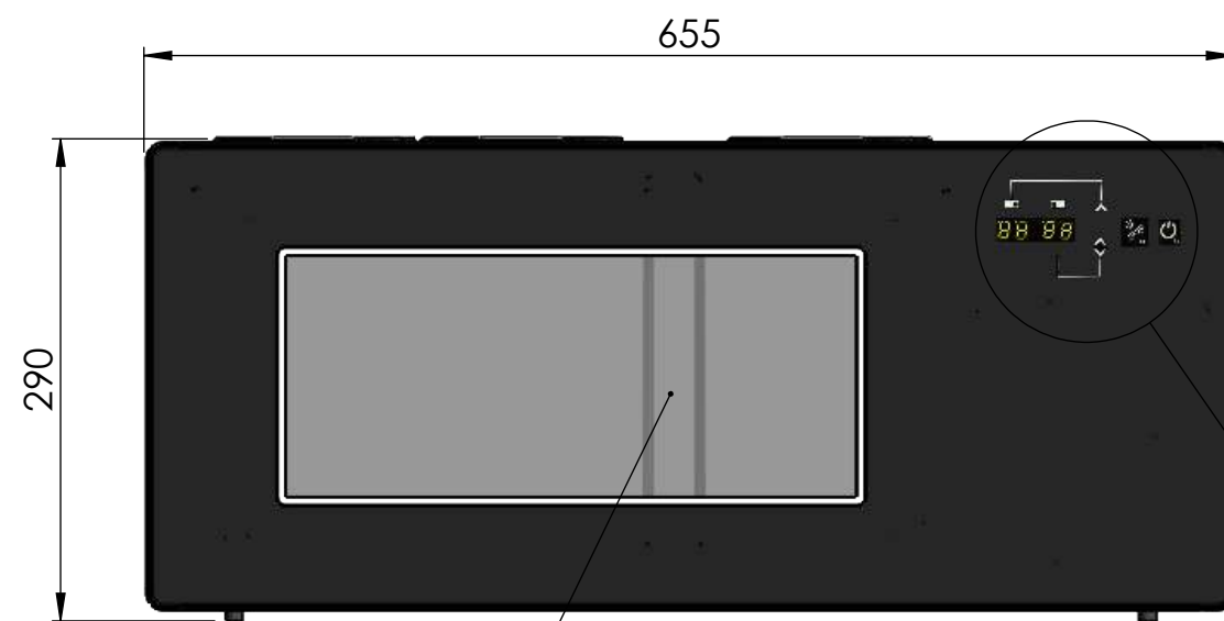
ALZADO
